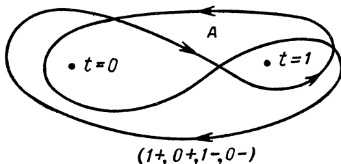
Рис. 4. Области сходимости.
