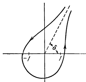
t -плоскость
