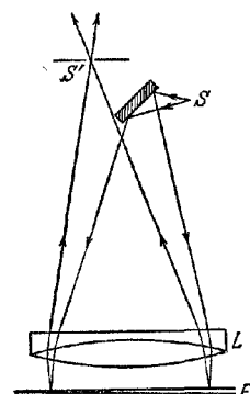
Рис. 7.30. Схема интерферометра Физо.
