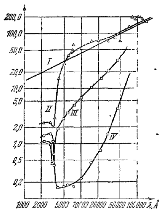
Рис. 13.3. Зависимость оптических постоянных серебра от длины волны. I — теоретическая кривая nk , II — экспериментальная кривая n(1 - \mathcal{R}) , III — экспериментальная кривая nk , IV — экспериментальная кривая n . Логарифмический масштаб
