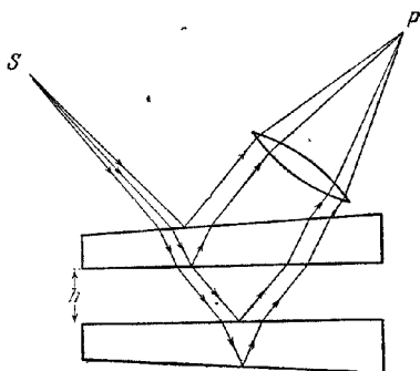
Рис. 7.22. Плоскопараллельная воздушная прослойка, возникновение полос, локализованных в бесконечности.
