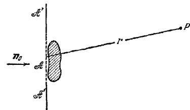
Рис. 13.12. К выводу соотношения (114) для сечения экстинкции при большом препятствии
