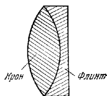
Рис. 4.25 Ахроматически дублет
