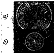
Рис. 9.4. Изображения в плоскости красного фокуса (а) и в плоскости геометрического круга наименьшего рассеяния (б) при наличии первичной сферической aberrации \Phi = 16\lambda\rho^4 [15]
