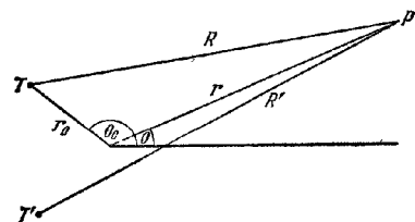
Рис. 11 16 Взаимное расположение линейного источника T и дифракционного экрана, занимающего полуплоскость.
