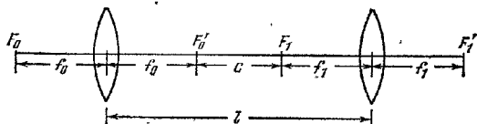
Рис. 4.16. Система из двух центрированных тонких линз.
