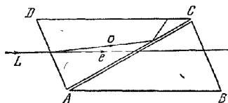
Рис. 14.17. Призма Николя.
