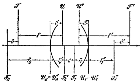
Рис. 4.14. Кардинальные точки комбинированной системы (толстая линза).
