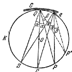
Рис. 8.26. Фокусировка в случае вогнутой решетки (круг Роулянда).
