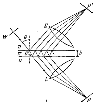
Рис. 7.57. К возникновению многолучевых интерференционных полей равного наклона в случае плоскопараллельной пластинки.
