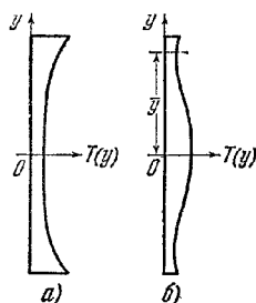
Рис. 6.21. Сечение корректирующей пластинки Шмидта.
