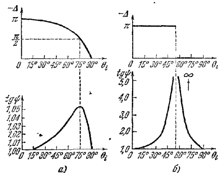
Рис. 13.2. Величины -\Delta = \varphi_{\perp} - \varphi_{\parallel} и P = \text{tg}\psi = -\rho_{\perp}/\rho_{\parallel} , характеризующие изменение состояния поляризации света при отражении от типичного металла (а) и прозрачного диэлектрика (б).
