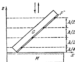
Рис. 7.18. Опыт Винера со стоячими волнами.
