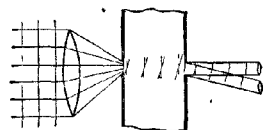
Рис. 14.16. Внешняя коническая рефракция.
