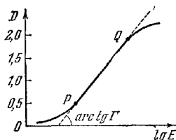
Рис. 8.49. Кривая Хертнера — Дриффельда (характеристическая кривая).
