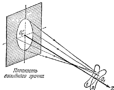
Рис 5.6. Тангенциальная и сагитальная фокальные поверхности.
