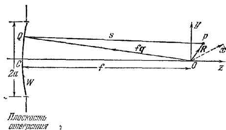
Рис. 8.38 К дифракции на круглом отверстии сходящейся сферической волны
