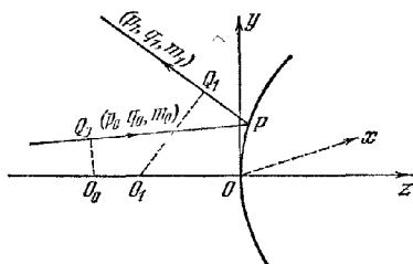
Рис 4.5 Угловая характеристика отражающей поверхности вращения. Точки O, O_1, O, Q_0, P, Q_1 не обязательно компланарны
