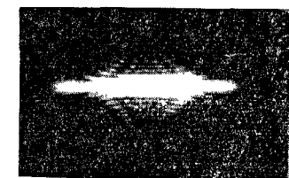
Рис. 9.11. Изображение в плоскости, в которой лежит фокальная линия, при наличии первичного астигматизма \Phi = 2,7\lambda\sigma^2 \cos 2\theta [15].
