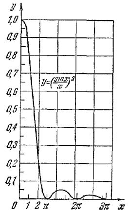
Рис. 8.9 Дифракция Фраунгофера на прямоугольном отверстии.
