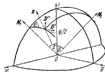
Рис. 14.29. К теории поглощающих кристаллов.
