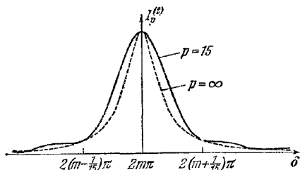
Рис 7.69. Зависимости интенсивности в интерференционных полосах, полученных с пластинкой Люммера — Герке, от разности фаз ( \mathcal{R} = 0,87 )
