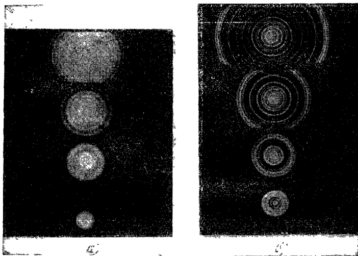
Рис. 9.5. Изображения в параксиальной фокальной плоскости (а) и в плоскости геометрического кружка наименьшего рассеяния (б) при наличии первичной сферической aberrации \Phi=17,5 \lambda \rho^4 ; 8,4 \lambda \rho^3 , 3,7 \lambda \rho^2 и 1,4 \lambda \rho [15]
