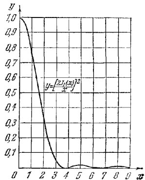
Рис. 8.11. Дифракция Фраунгофера на круглом отверстии.
