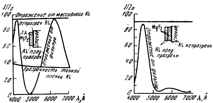
Рис. 17.6. Типичная спектральная характеристика простейшего отражательного фильтра
