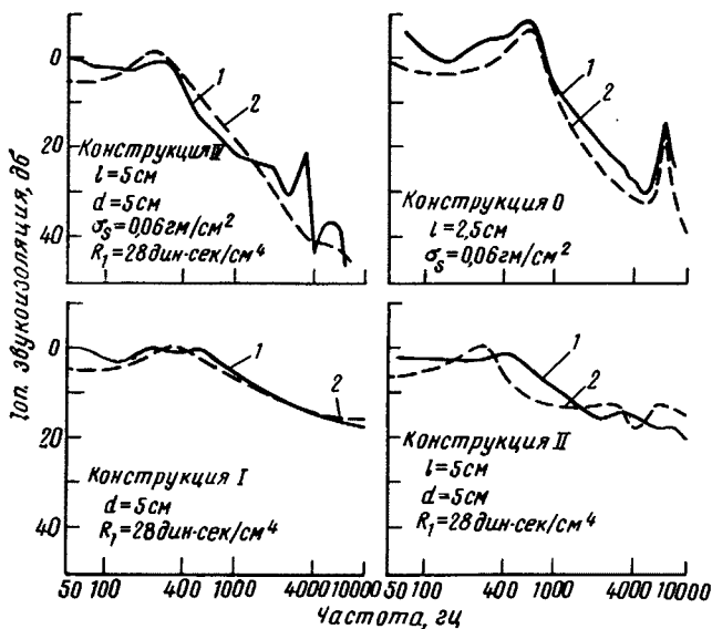
Рис. 18.5. Сравнение экспериментальных и теоретических данных для звукоизоляции различных конструкций в зависимости от частоты. По оси ординат — превышение звукоизоляции данной конструкции по сравнению со звукоизоляцией одиночной стенки с плотностью \sigma_1/\text{см}^2
