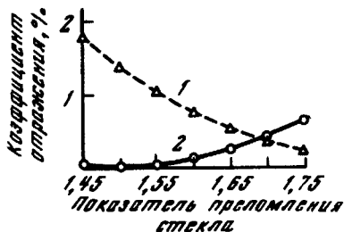
Рис. 16.4. Влияние величины показателя преломления внутреннего слоя при двухслойном просветлении стекла на значение минимального коэффициента отражения, осуществляющегося при четвертьволновых слоях. Показатель преломления верхнего слоя 1,47, стекла 1,525
