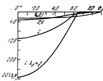
Рис. 20.6. Коэффициент отражения волны от симметричного слоя в зависимости от угла падения для различных толщин слоя n_1 = 0,9
