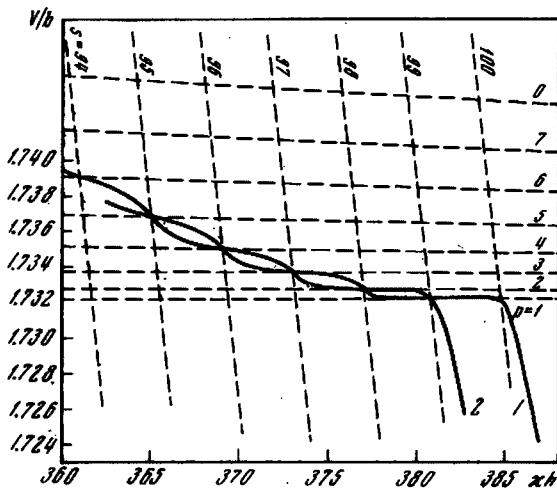
Рис. 9.8. Кривые фазовых скоростей для симметричной (1) и антисимметричной (2) волн ( l = 50 , \sigma = 0,25 )
