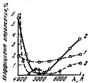
Рис. 16.14. Спектральные характеристики типичных одно-, двух- и трехслойного покрытий (кривая 1), двухслойного (кривая 2) и трехслойного (кривая 3) покрытий
