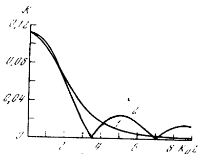
Рис. 20.4. Сравнение коэффициентов отражения в функции толщины слоя для двух видов переходных слоев, показатель преломления для которых изображен на рис. 20.5;
