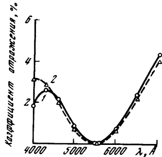
Рис. 16.8. Теоретическая спектральная характеристика двухслойного покрытия
