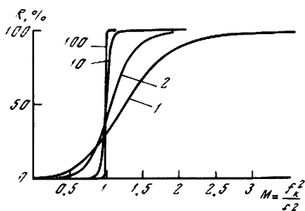
Рис. 20.8. Зависимость коэффициента отражения R = \rho^2 по энергии от частоты для простейшего ионосферного слоя для различных толщин слоя
