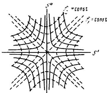
Рис. 27.1. Окрестность точки перевала
