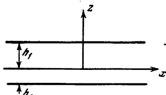
Рис. 12.1. К теории распространения звука в мелкослойной среде
