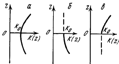
Рис. 47.1. К определению коэффициента отражения от нижнего и верхнего неоднородных полупространств
