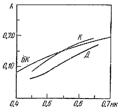
Рис. 9. Кривые спектральной отражательной способности «морей» Марса: БК — Н. П. Барабанов и И. К. Коваль, К — И. К. Коваль, Д — О. Дольфус.
