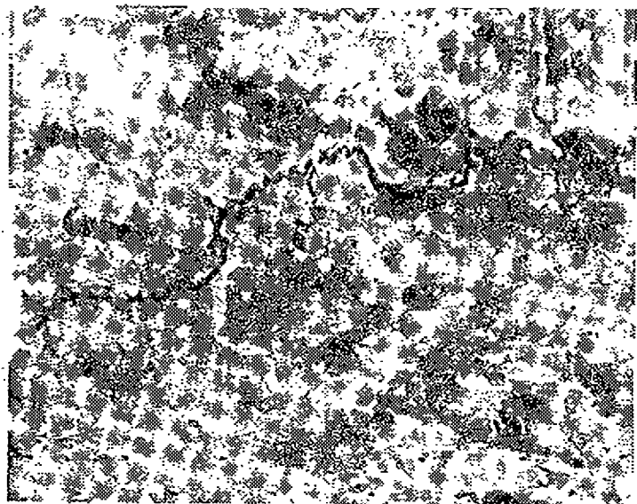
Рис. 17. Руслоподобные протоки на Марсе.
