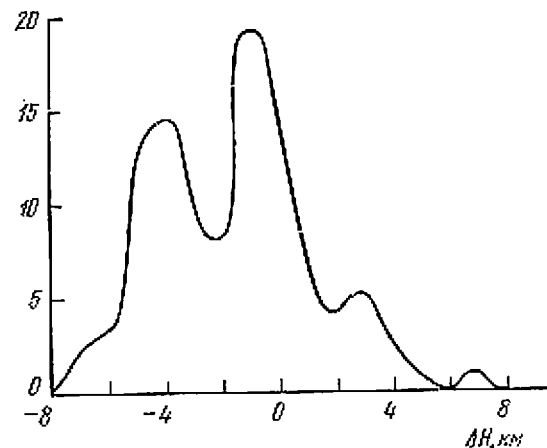
Рис. 18. Гипсометрическая кривая для Марса, показывающая частоту встречаемости уровней высот (от условного нуля).
