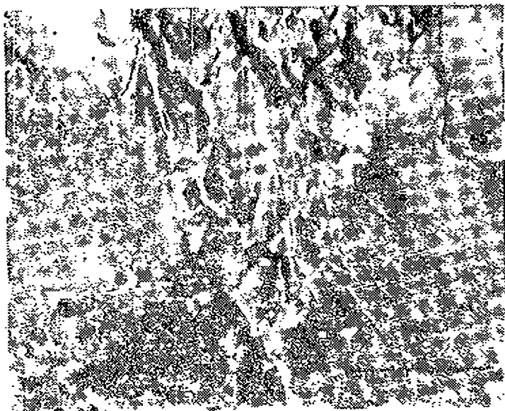
Рис. 16. Система разломов «Люстра», примыкающая к гребню Коэрат. Снимок «Маринера-9».
