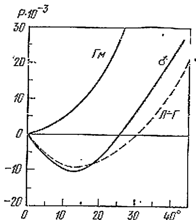
Рис. 10. Поляризационные кривые для материков Марса ( \sigma ) и порошков минералов, Гм — гематит, П+Г — смесь лимонита и гетита (по О. Дольфюсу).
