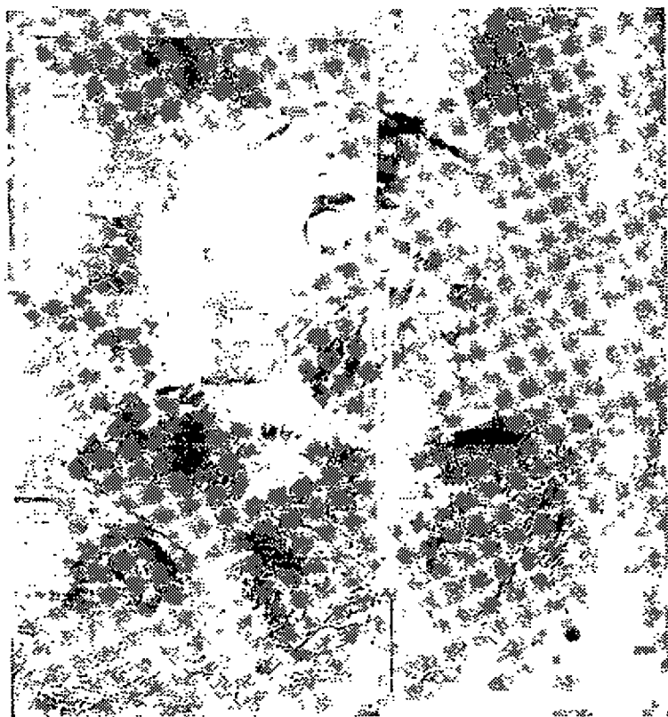
Рис. 13. Верхняя кальдера Nix Olympica — самая высокая гора на Марсе.
