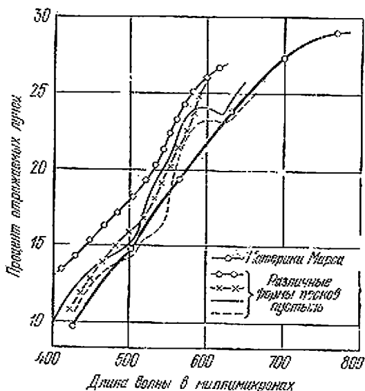
Рис. 8. Кривые спектральной отражательной способности материалов Марса и песков земных пустынь (по Н. И. Сизинскому и Е. Л. Кризову).
