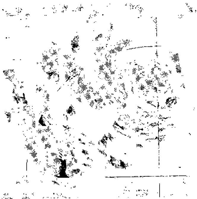
Рис. 22. Слоистая структура полярной шапки Марса (по снимкам «Маринера-9»).
