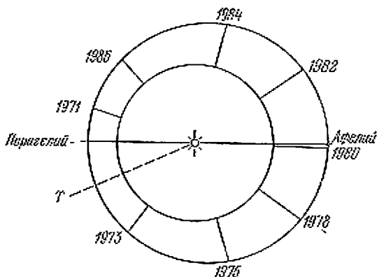
Рис. 1. Орбиты Марса и Земли. Указаны годы противостояний Марса.
