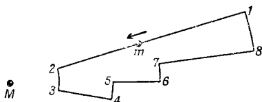
Ф и г. 13.3. Замкнутый путь обхода в поле тяготения.
