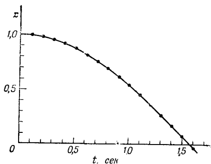
Ф и г. 9.1. График движения грузика на пружинке.
