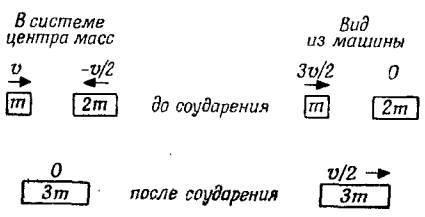
Ф и г. 10.7. Неупругое соударение между телами с массами m и 2m .
