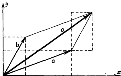
Ф и г. 11.4. Сложение векторов.
