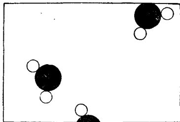
Ф и г. 1.2. Пар под микроскопом.
