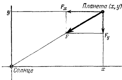
Ф и г. 9.5. Сила притяжения, действующая на планету.
