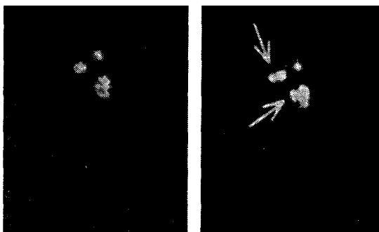
Ф и г. 7.12. Образование новых звезд?
