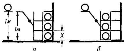
Фиг. 4.2. Обратимая машина. a — начальное положение; б — загрузка шаров; в — 1 кг поднимает 3 кг на высоту X ; г — разгрузка шаров; д — восстановление; е — конечное положение.
