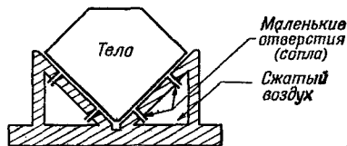
Фиг. 10.1. Воздушный желоб (вид с торца).
