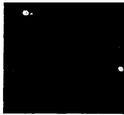
Ф и г. 7. в. Система двойной звезды.
