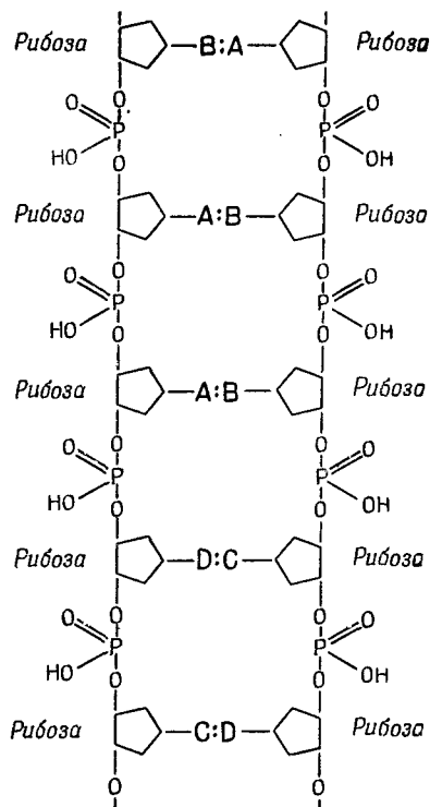
Ф и г. 3.2. Схема ДНК.
