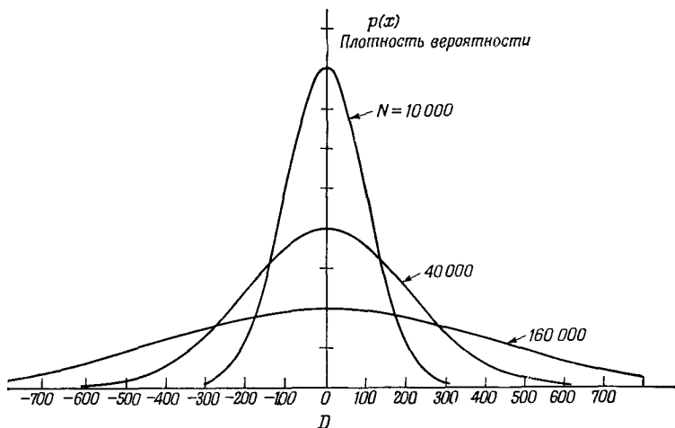
Ф и г. 6.7. Плотность вероятности окажется при случайном блуждании через N шагов на расстоянии D .
