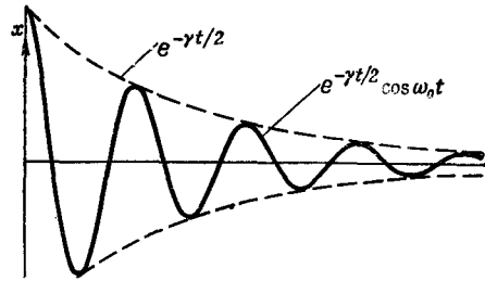
Ф и г. 24.1. Затухающие колебания.
