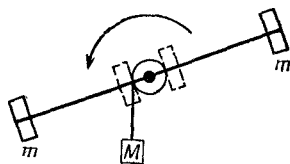
Ф и г. 18.4. Зависимость «инерции вращения» от плеча масс.
