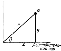
Ф и г. 23.1. Комплексное число, изображенное точкой на «комплексной плоскости».
