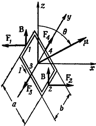
Фиг. 15.1. Прямоугольная петля с током I в однородном поле B , направленном по оси z .
