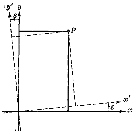
Ф и г. 18.2. Поворот осей во- круг оси z на малый угол \varepsilon .
