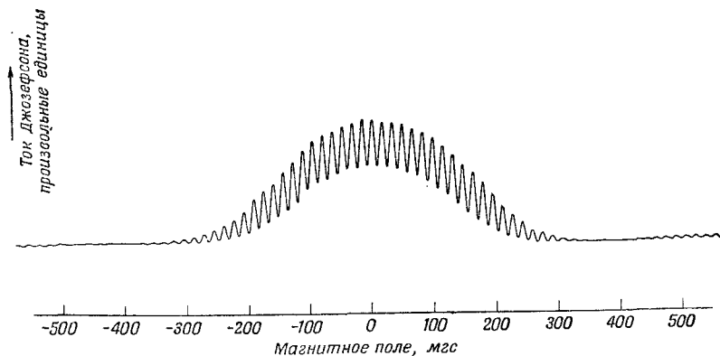
Ф и г. 19.8. Запись тока через два параллельных перехода Джозефсона как функции магнитного поля в области между двумя переходами.
