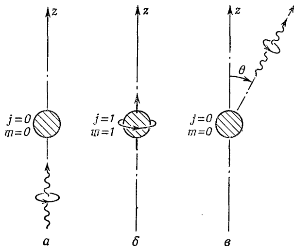
Ф и г. 16.4. Рассеяние света атомом, рассматриваемое как процесс, состоящий из двух шагов.
