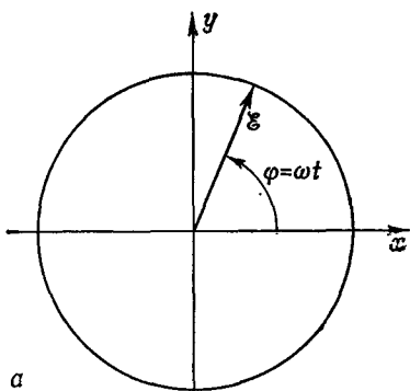
Фиг. 15.5. Электрическое поле \mathcal{E} в поляризованной по кругу световой волне (а) и вращение электрона, приводимого в движение поляризованным по кругу светом (б).
