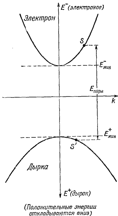
Ф и г. 12.4. Энергетические диаграммы для электрона и дырки.
