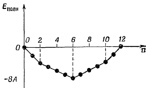
Ф и г. 13.13. Сумма всех энергий электронов, когда нижние состояния на фиг. 13.8 заполнены n электронами (принято E_0 = 0 ).
