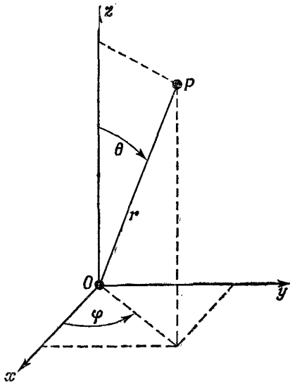
Фиг. 17.1. Сферические координаты r, \theta, \varphi точки P .
