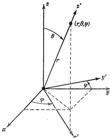
Фиг. 17.3. Точка (x, y, z) лежит на оси z' системы координат x', y', z' .
