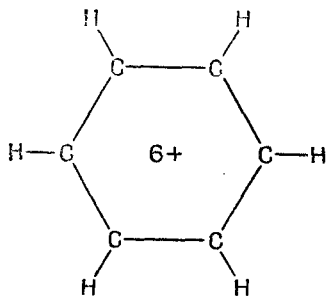
Ф и г. 13.4. Бензольное кольцо, из которого убрали шесть электронов.
