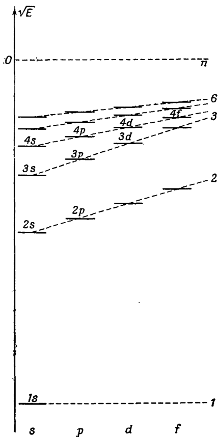
Ф и г. 17.8. Схематическая диаграмма уровней энергии атомного электрона в присутствии других электронов.
