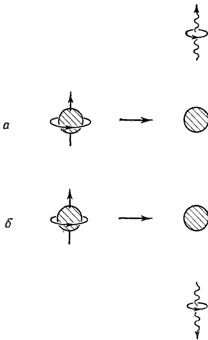
Ф и г. 16.3. Если процесс (а) преобразовать путем инверсии относительно центра атома, он станет выглядеть, как (б).
