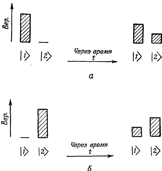
Фиг. 15.2. Если в симметричной системе чистое состояние |1\rangle развивается во времени так, как показано в части (а), то чистое состояние |2\rangle будет во времени развиваться так, как показано в части (б).
