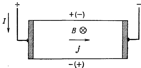
Ф и г. 12.6. Эффект Холла возникает при действии магнитных сил на носители.
