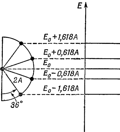
Ф и г. 13.11. Энергетические уровни бутадиена.
