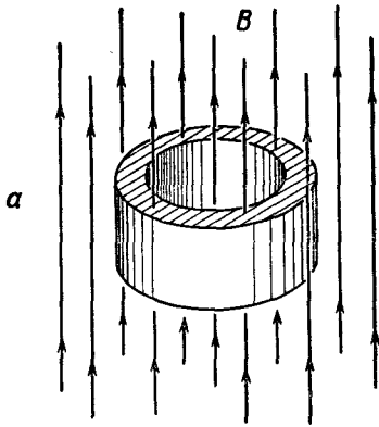
Ф и г. 19.4. Кольцо в магнитном поле.
