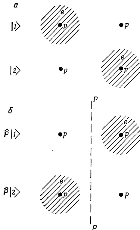
Ф и г. 15.1. Если состояния |1\rangle и |2\rangle отразить в плоскости P-P , они перейдут соответственно в состояния |2\rangle и |1\rangle .
