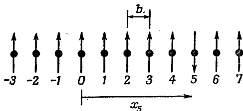
Ф и г. 13.1. Базисное состояние |x_5\rangle системы спинов, расположенных по одной линии.
