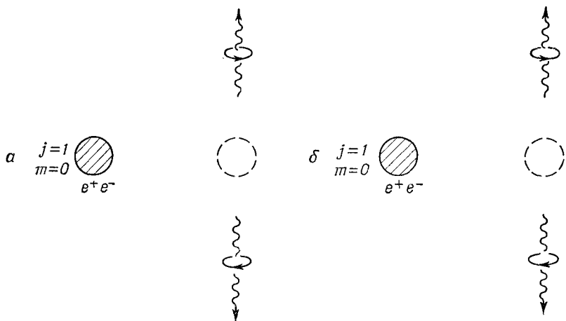
Фиг. 16.7. Для состояния позитрония с j = 1 процесс (а) и процесс (б), получаемый поворотом (а) вокруг оси y на 180^\circ , в точности совпадают.
