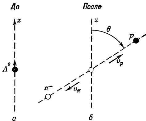
Ф и г. 15.6. \Lambda^0 -частица со спином, направленным вверх, распадается на протон и пион (в системе центра масс).
