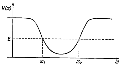
Фиг. 14.3. Потенциальная яма для частицы, движущейся вдоль оси x .
