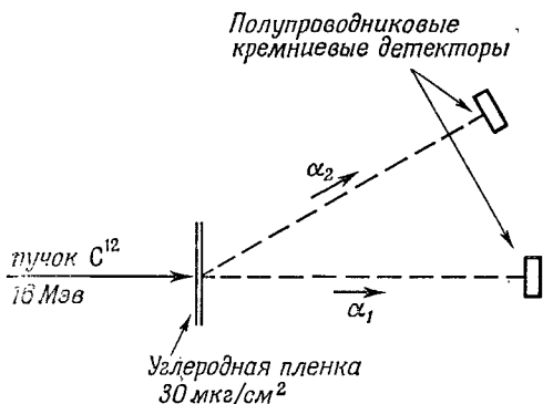
Ф и г. 16.9. Размещение приборов в опыте по определению спина возбужденных состояний Ne^{20} .
