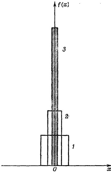
Ф и г. 14.2. Последовательность функций, ограничивающих единичную площадь, вид которых все сильнее и сильнее напоминает \delta -функцию.
