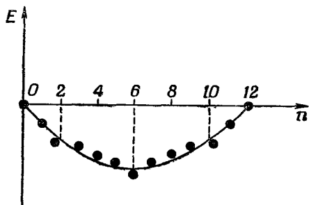
Ф и г. 13.14. Точки с фиг. 13.13 и плавная кривая. Молекулы с n=2, 6, 10 устойчивее остальных.
