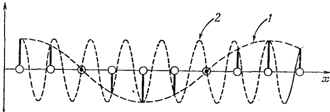
Фиг. 11.4. Пара значений k , представляющих одну и ту же физическую ситуацию.
