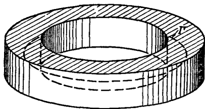
Фиг. 19.5. Кривая \Gamma внутри сверхпроводящего кольца.
