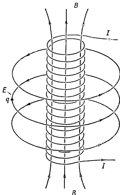
Ф и г. 19.2. Электрическое поле снаружи соленоида, ток в котором увеличивается.
