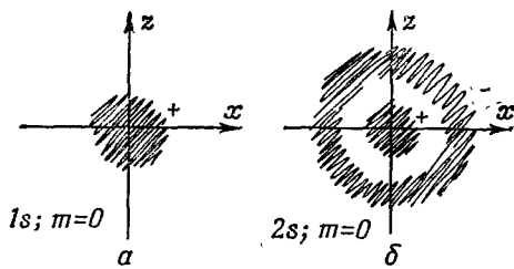
Ф и г. 17.6. Наброски, отражающие общий характер волновых функций водорода.
