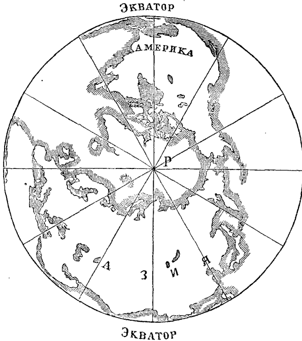
Фиг. 22. Вид земного шара с точки над полюсом Р.
