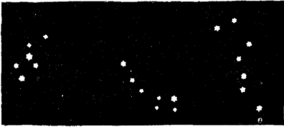
Фиг. 84. Кассиопея , Малая Медведица с Полярной звездой, Большая Медведица .
