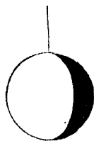
Фиг. 43. 6-е положение. Темная сторона показывается узкою полоскою справа.
