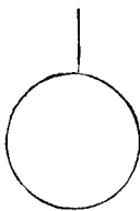
Фиг. 42. 5-е положение. Освещенная сторона видна вполне.
