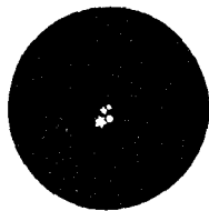
Фиг. 92. Вид четверной звезды в телескопе.
