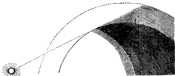
Фиг. 19. Сумерки. Верхние слои атмосферы еще освещены пад частью поверхности Земли, уже находящейся в тени.
