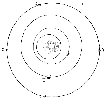
Фиг. 70. Орбита Марса и его положение относительно Земли T . Две другие, ближайšie к Солнцу планеты — Венера и Меркурий.
