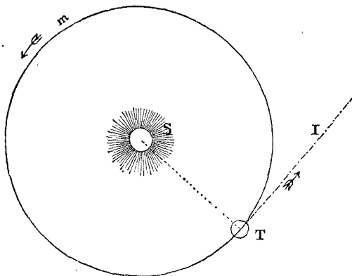
Фиг. 61. Т — Земля; S — Солнце; TI — путь, по которому пошла бы Земля, если бы Солнце не притягивало ее к себе по направлению TS.
