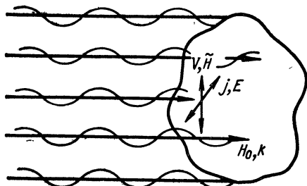
Рис. 11. Структура волны с круговой поляризацией.
