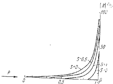
Рис. 18,4. Коэффициент отражения для «переходного» слоя.
