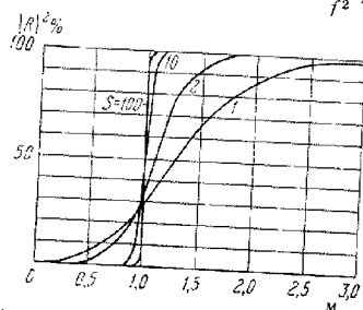
Рис. 18,3. Коэффициент отражения для «симметричного» слоя.
