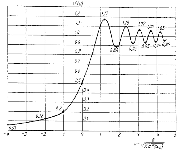
Рис. 21.1. Форма переднего края импульса, который до прохождения среды был прямоугольным.
