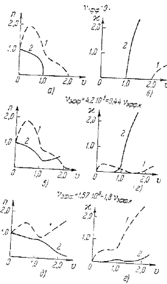
Рис. 11,14. Показатели преломления и поглощения для \lambda = 225 м и различных значений \nu_{эфф} (значения a и u указаны в тексте).
