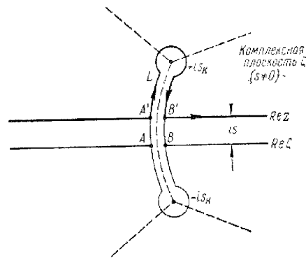
Рис. 28,9. Контур интегрирования в выражении (28,53).
