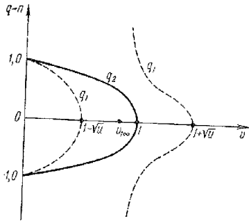
Рис. 29,1. Функции q_{1,2}(v) при нормальном падении ( \mu = \frac{1}{4} , \alpha = 45^\circ ).
