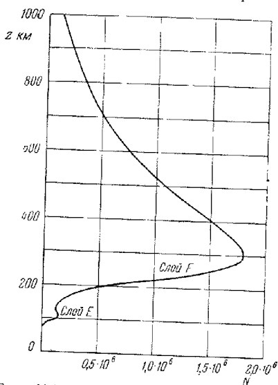
Рис. 30.1. Электронная концентрация N в ионосфере (средние широты, полдень, годы максимума солнечной активности; приводятся некоторые усредненные значения).
