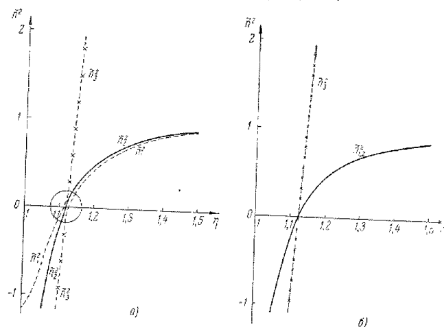
Рис. 36.7. Функции \tilde{n}_{1,2,3}^2 в корональной плазме при \alpha = 15^\circ : а) H_b = 25 эрст; б) H_b = 0 (изотропная плазма).
