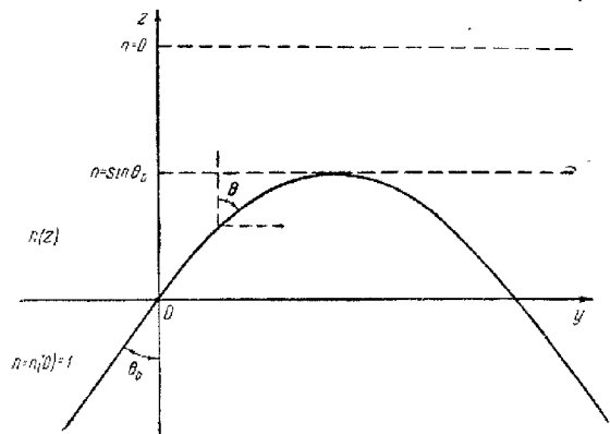
Рис. 19,1. Наклонное падение волн на слой. При z < 0 показатель преломления равен n = n(0) = 1 , при z > 0 он равен n = n(z) .
