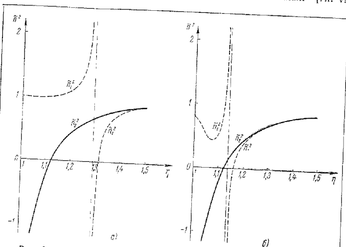
Рис. 36.6. Функции \tilde{n}_{1,2}^2(\eta) в корональной плазме при \alpha = 90^\circ : а) H_b = 2,5 \cdot 10^3 ; б) H_b = 2,5 \cdot 10^2 .
