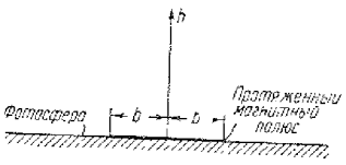
Рис. 36,3. Протяженный магнитный полюс, имеющий форму окружности с радиусом b и находящийся на уровне фотосферы.
