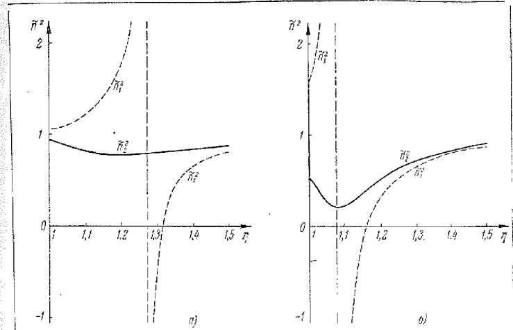
Рис. 36,4. Функции \tilde{n}_{1,2}^2(\eta) в корональной плазме при \alpha = 0 (вертикальные пунктирные линии отвечают точке \nu_{100} ): a ) H_b = 2,5 \cdot 10^3 ; b ) H_b = 2,5 \cdot 10^2 .
