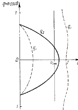
Рис. 29,3. Функции q_{1,2}(v) для распространения на экваторе в плоскости магнитного меридиана ( \theta_0 = 42^\circ , \mu = \frac{1}{4} ).
