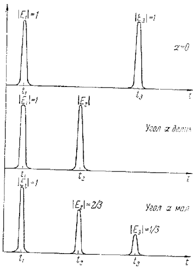
Рис. 28.2. Эффект «утраивания» отраженных сигналов при u < 1 и разных углах \alpha (схематически).
