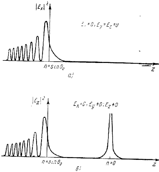
Рис. 20,1. Квадрат модуля компоненты электрического поля при отражении от неоднородного слоя волны, падающей под углом \theta_0 . Показатель преломления равен n = n(z) : а — волна с электрическим вектором, перпендикулярным к плоскости падения; б — волна с электрическим вектором, лежащим в плоскости падения.
