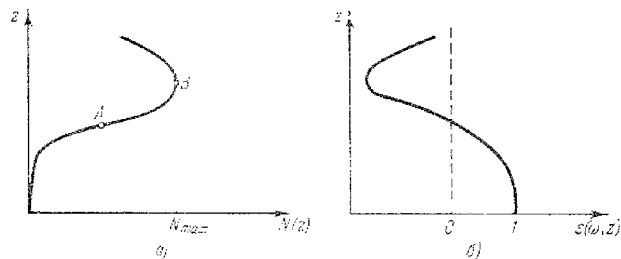
Рис. 30,4. Произвольный плавный слой с одним максимумом.
