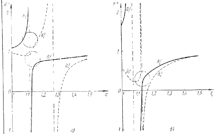
Рис. 36,5. Функции \tilde{n}_{1,2}^2(\eta) в корональной плазме при \alpha = 15^\circ (вертикальные пунктирные линии отвечают точкам \nu_{100} и \nu_{200} ): a ) H_b = 2,5 \cdot 10^3 ; b ) H_b = 2,5 \cdot 10^2 .
