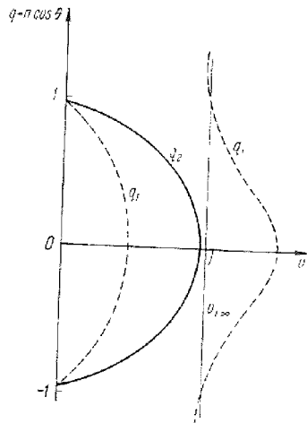
Рис. 29,2. Функции q_{1,2}(v) для распространения на полюсе (вертикальное магнитное поле H^{(0)} ). Используются значения \theta_0 = 20^\circ , \mu = \frac{1}{4} .
