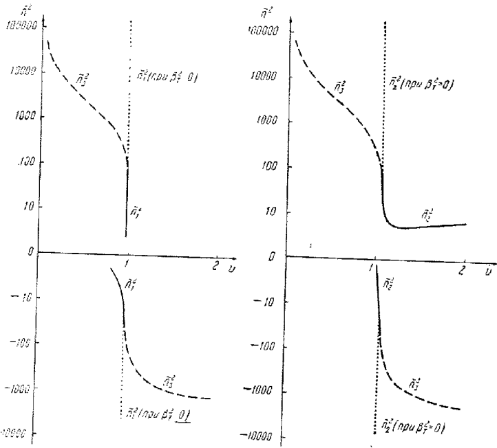
Рис. 12.11. Функции \tilde{n}_1^2 и \tilde{n}_3^2 при u = 0,5, \alpha = 10^\circ и \beta_T^2 = 10^{-4} . Рис. 12.12. Функции \tilde{n}_1^2 и \tilde{n}_3^2 при u = 2, \alpha = 10^\circ и \beta_T^2 = 10^{-4} .
