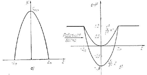
Рис 17,2. Параболический слой: а) N(z) ; б) \epsilon(z) при \frac{f_k^2}{f^2} = 1 и \frac{f_k^2}{f^2} = 2 .
