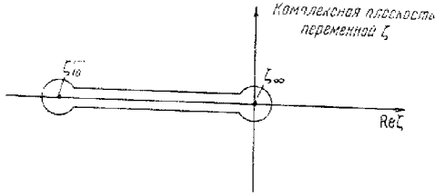
Рис. 27,4. Контур интегрирования в выражении (27,17), причем контур нужно обойти два раза (двулиственный характер поверхности на рисунке не отражен).
