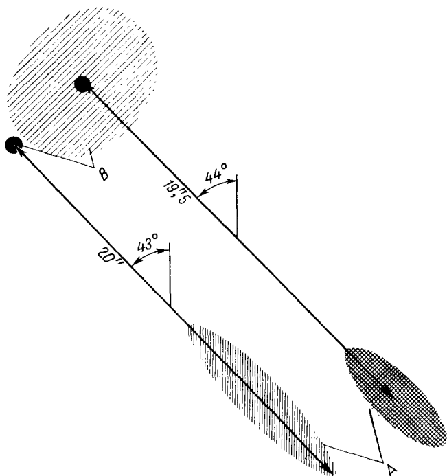
Рис. 5. Структура источника 3С 273, определенная М. Шмидтом по паломарским фотографиям (слева), очень близка к тому, что получено по лунному покрытию этого источника (справа).
