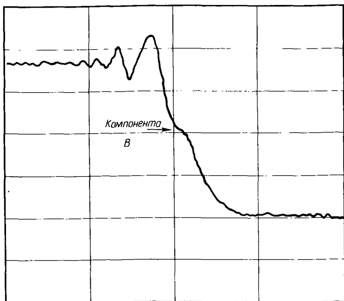
Рис. 4. Покрытие радиисточника Луной позволяет с высокой точностью определить его положение и строение. На кривой видно, как радиосигнал от двухкомпонентной сверхзвезды ЗС 273 был прерван Луной 5 августа 1962 г.; запись принадлежит австралийским наблюдателям, работавшим с 70-метровым радиоте-
