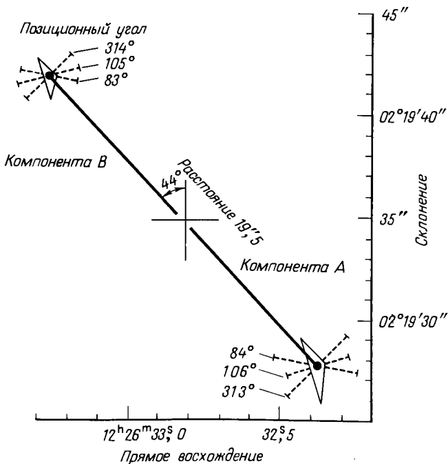
Рис. 4. Схема радиисточника 3С 273. Стороны треугольников изображают положения краев Луны во время покрытия. Пуиктириыми линиями показана эквивалентная ширина источника на частоте 410 Мгц для каждого из трех позиционных углов, отмеченных на схеме.
