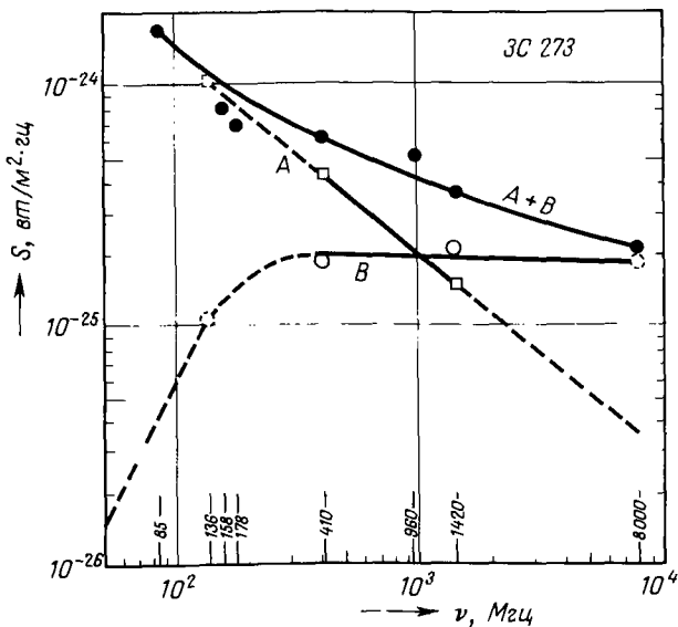
Рис. 6. Радиоспектр 3C 273. Линия, проведенная через светлые кружки (компонента B), показывает, как можно подогнать эти данные под тепловой спектр. Однако вся эта интерпретация представляется не слишком правдоподобной.
