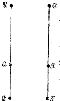
Фиг. 4. \mathbb{K} —группа характеров группы \mathbb{A}/\mathbb{U} ; \mathbb{K} \cong \mathbb{A}/\mathbb{U} . \mathbb{X}/\mathbb{K} —группа характеров группы \mathbb{U} ; \mathbb{X}/\mathbb{K} \cong \mathbb{U}
