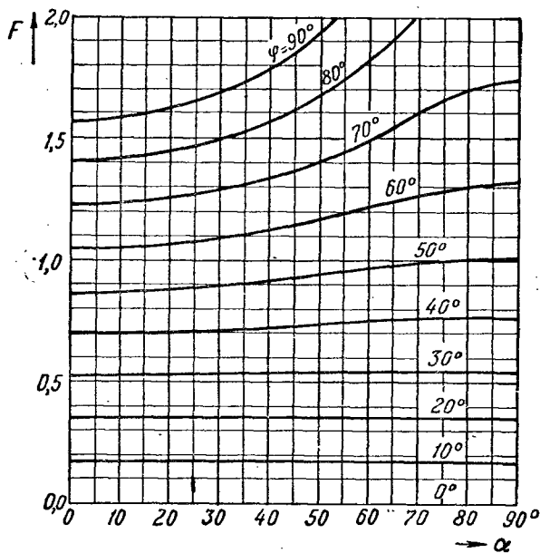
Рис. 44. Кривые F(\varphi, \sin \alpha) , \varphi = \text{const.}
