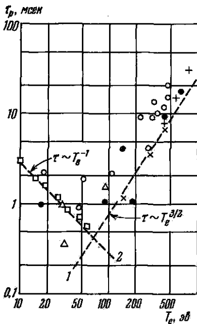
Рис. 32.15. Время жизни частиц в зависимости от электронной температуры. 1) Токамак ST; B_{||} = 43 кГс; прямая проведена через нижние точки. Обозначения +, O, ●, × и Δ соответствуют диаметрам диафрагм 130, 120, 80, 60 и 40 мм. 2) Стелларатор-С; B_{||} = 11 кГс; прямая отвечает расчетному времени жизни по Бому; □ — экспериментальные точки, диаметр диафрагмы 50 мм.
