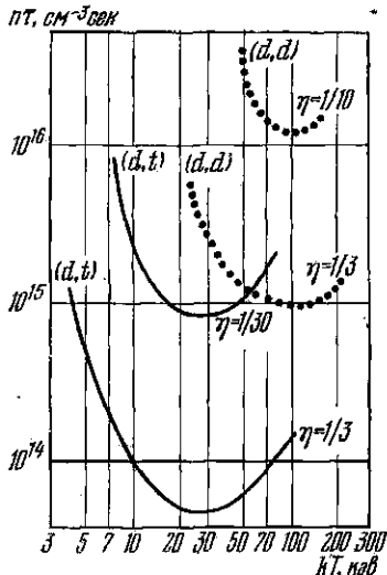
Рис. 4.2. Критерий Лоусона для реакций (d, t) и (d, d) при различных значениях к. п. д. реактора.
