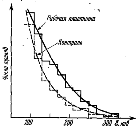
Рис. 35.11. Гистограмма распределения электронов по энергиям, полученная при обработке 1500 треков в ядерной эмульсии, защищенной 20 мк Рб.
