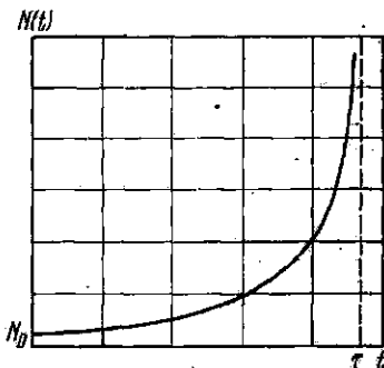
Рис. 38.2. Программированное выделение мощности для получения сверхжаркого состояния.
