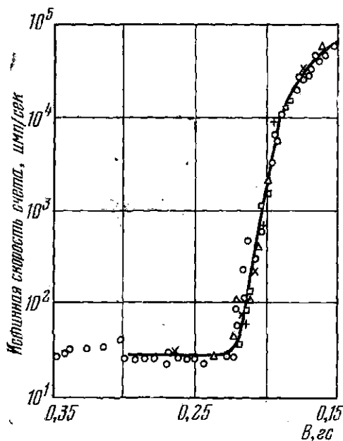
Рис. 7.2. Зависимость скорости счета от напряженности геомагнитного поля. (○ — результаты, полученные при полете спутника над Азией; □, × — над Африкой; Δ, + — над Южной Америкой.)
