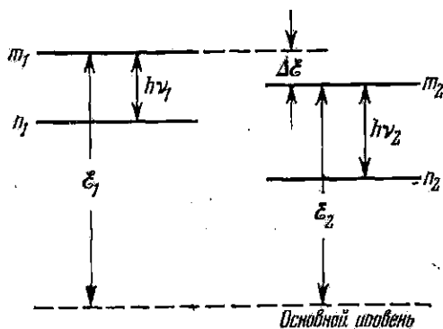
Рис. 22.1. Схема энергетических термов.
