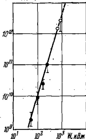
Рис. 37.9. Зависимость нейтронного выхода от энергосодержания. ● и ○ — соответственно опыты 1970 г. и 1973 г.
