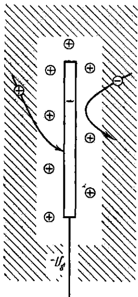
Рис. 18.3. Картина распределения зарядов в плазме при отрицательном потенциале на зонде.
