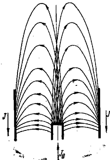
Рис. 37.6. «Фонтанирующий пинч». Положение фронта тока в последовательные моменты времени.
