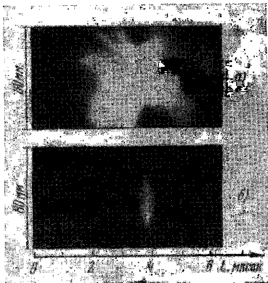
Рис. 34.14. Временная развертка свечения плазмы Z-пинча в спектрально разложенном свете: а) для спектрального интервала в области H_\alpha ( \Delta\lambda = 100 \text{ \AA} ); б) в области \lambda = 6400 \text{ \AA} ( \Delta\lambda = 100 \text{ \AA} , континуум). Начальное давление 0,1 тор.
