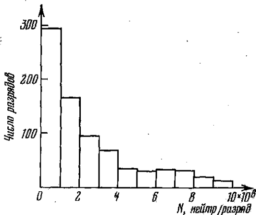
Рис. 35.1. Гистограмма распределения числа разрядов по интенсивности нейтронного выхода. N —число нейтронов за разряд. U_0 = 30 кВ, P_0 = 6 \times 10^{-2} тор. Обработано 900 экспериментов.
