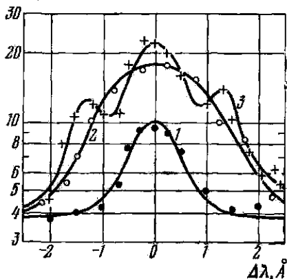
Рис. 21.8. Профиль линии H_{\beta} для трех моментов времени: 1 — перед ударной волной, 2 — на фронте волны, 3 — позади фронта.
