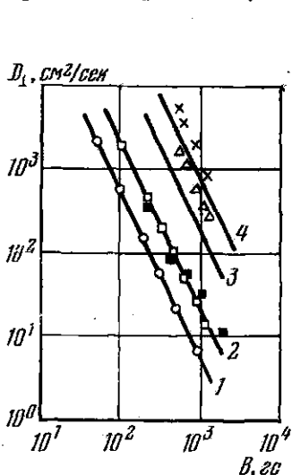
Рис. 11.3. Зависимость коэффициента поперечной диффузии в гелиевой плазме от магнитного поля для нескольких значений электронной плотности. 1) n_e < 10^9 \text{ см}^{-3} ; 2) n_e < 10^{10} \text{ см}^{-3} ; 3) n_e = 2,7 \times 10^{11} \text{ см}^{-3} ; 4) n_e \approx 10^{12} \text{ см}^{-3} .
