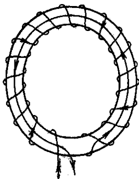
Рис. 17.2. Пояс Роговского с обратным витком, компенсирующим магнитный поток через отверстие тора.
