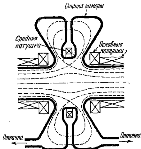
Рис. 33.9. Схема устройства дивертора.
