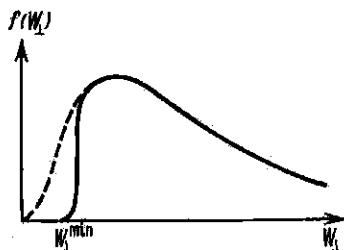
Рис. 30.12. Деформация функции распределения частиц по поперечной энергии при возрастании потенциала плазмы.
