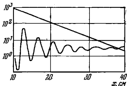
Рис. 12.4. Результаты измерения затухания Ландау.
