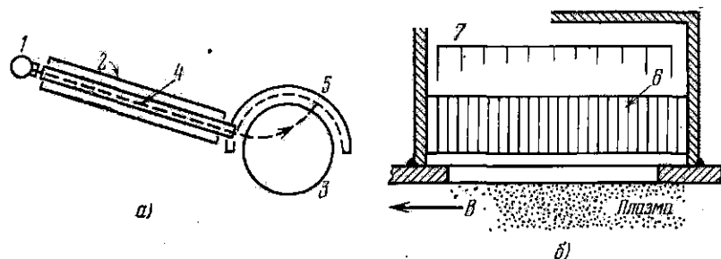
Рис. 26.3. Схема измерительного устройства, используемого для изучения потенциала плазмы (а), и детали детектора (б). 1 — источник ионов SF_6^- ; 2 — магнитный экран; 3 — камера с плазмой; 4 — ионный пучок; 5 — детектор ионов (регистратор пролетных времен); 6 — экранирующая решетка для подавления шумов от плазмы; 7 — приемный электрод.
