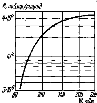
Рис. 35.3. Зависимость нейтронного выхода от подводимой мощности.
