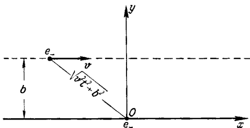
Рис. 14. Ионизационные потери.
