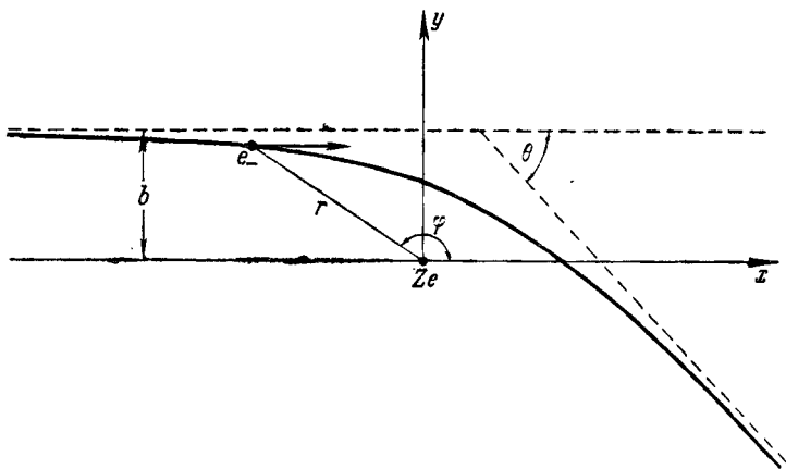
Рис. 11. Рассеяние быстрого электрона ядром.
