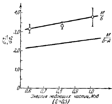
Рис. 28. Сравнение рассеяния электрона на электроне и позитрона на электроне.
