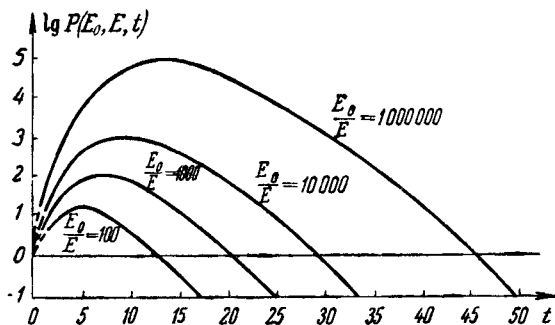
Рис. 20. Интегральный спектр электронов.
