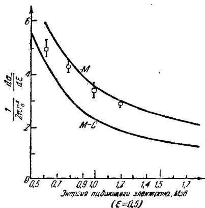
Рис. 26. Рассеяние электрона на электроном.
