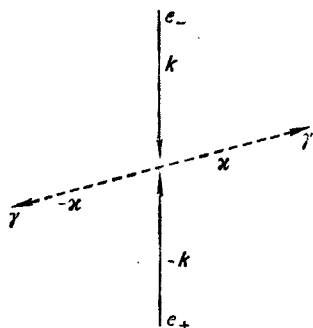
Рис. 17. Аннигиляция пары.
