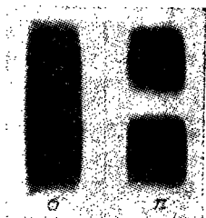
Рис. 6. Фотография \sigma - и \pi -компонент излучения «светящегося» электрона.
