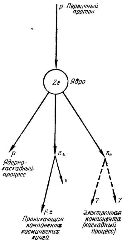
Рис. 18. Схема образования вторичной компоненты космических лучей.
