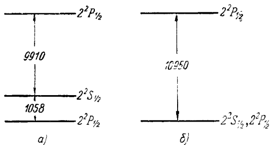
Рис. 24. Расположение термов в атоме водорода:
