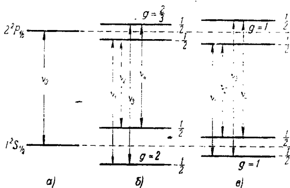
Рис. 25. Эффект Зеемана:
