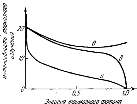
Рис. 13. Тормозное излучение.
