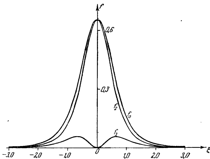
Рис. 2. Линейная поляризация в зависимости от угла излучения.
