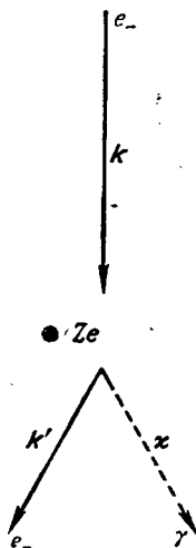
Рис. 12. Тормозное излучение.
