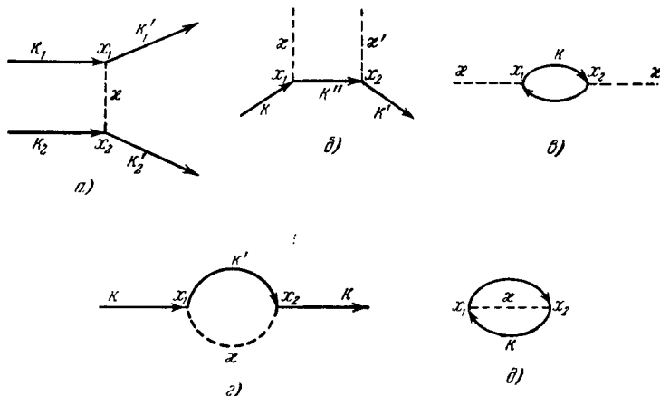
Рис. 21. Графики Фейнмана для различных процессов второго порядка.
