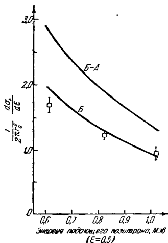
Рис. 27. Рассеяние позитрона на электроном.
