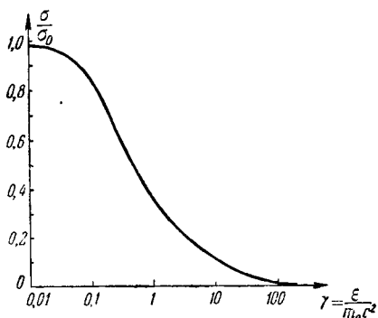
Рис. 10. Рассеяние \gamma -квантов свободными электронами.
