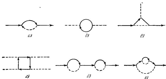
Рис. 22. Неприводимые и приводимые графики Фейнмана.
