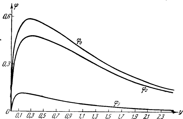
Рис. 4. Линейная поляризация в зависимости от частоты излучения.
