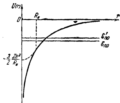
Рис. 29. Изменение потенциала в мезоатоме. Сплошная линия — потенциал точечного заряда. Пунктирная линия — учет конечных размеров ядра, сказывающихся при r < R_N , \epsilon_{no} — уровень энергии мезоатома при наличии точечного взаимодействия, \epsilon'_{no} — при учете конечных размеров ядра.
