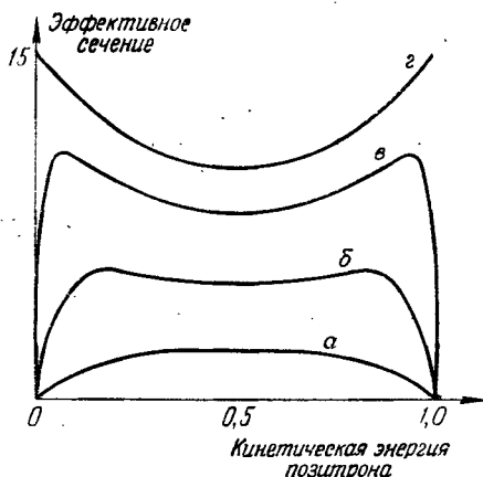
Рис. 16. Распределение пар по энергиям
