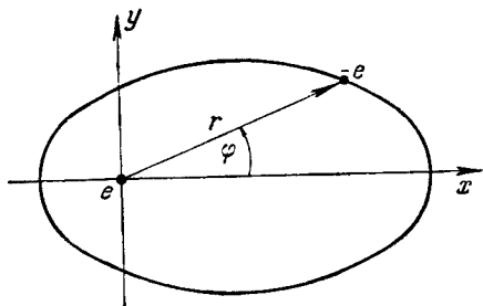
Рис. 23. Движение электрона в атоме водорода.
