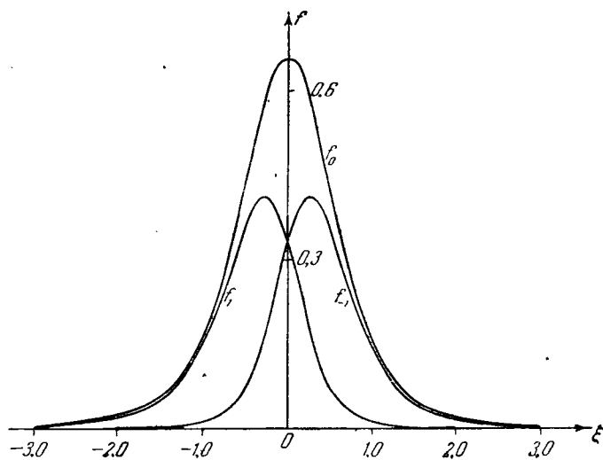
Рис. 3. Круговая поляризация в зависимости от угла излучения.
