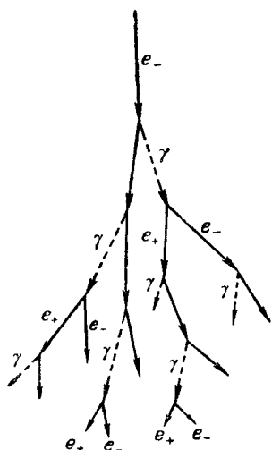
Рис. 19. Схема каскадного размножения электронной компоненты.
