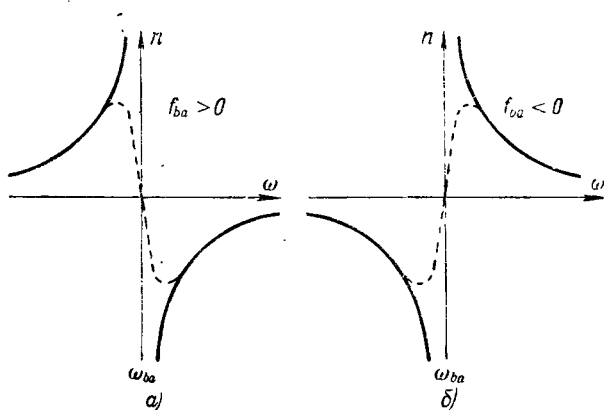
Рис. 8. Кривая дисперсии:
