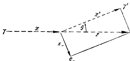
Рис. 9. Эффект Комптона.
