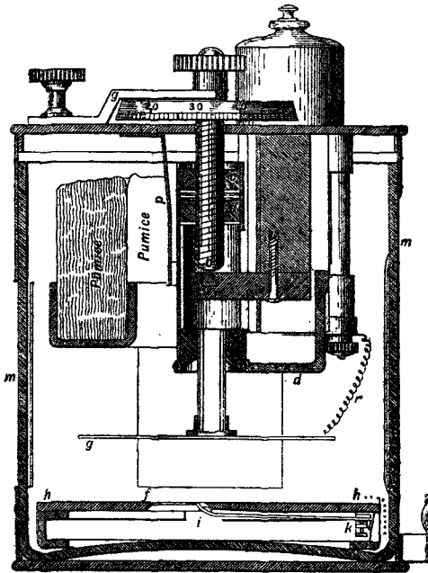
Рис. 56. —Переносный электрометръ, нынѣшній образецъ: \frac{2}{3} настоящей величины. [Pumice=пемза].
