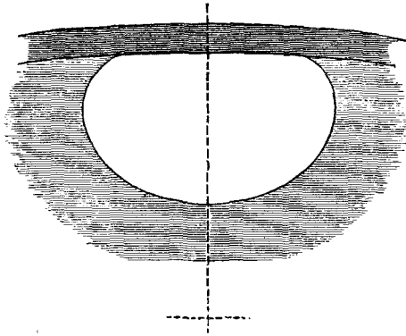
Рис. 27. Сѣченіе пузыря, воздуха въ трубкѣ уровня, наполненной водой и согнутой такъ, что ея ось есть часть окружности большаго радіуса: масштаб изображенъ на рис. 28.
