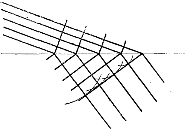
Рис. 35. Чертежъ построенія Гюйгенса для передней части волны преломленнаго свѣта; нарисованъ для свѣта, проходящаго изъ воздуха въ флинтгласъ.
