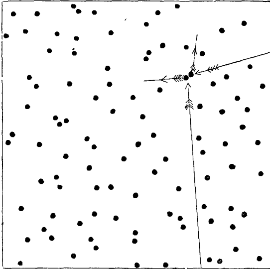
Рис. 43. Чертежъ, иллюстрирующий число молекулъ въ пространствѣ въ \frac{1}{10,000} сантиметра въ квадратъ и въ \frac{1}{100,000,000} сантиметра толщиной 1) .
