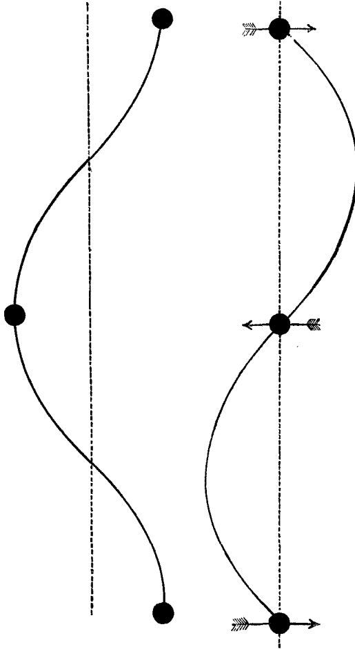
Рис. 40. Рис. 41. Двѣ частицы въ длинѣ одной волны.
