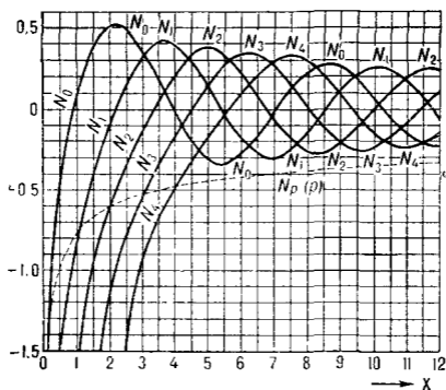
Графики функций Неймана.
